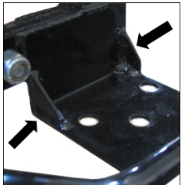
Ohjaushammastangon kiinnityslevyn lisävahvikkeet
