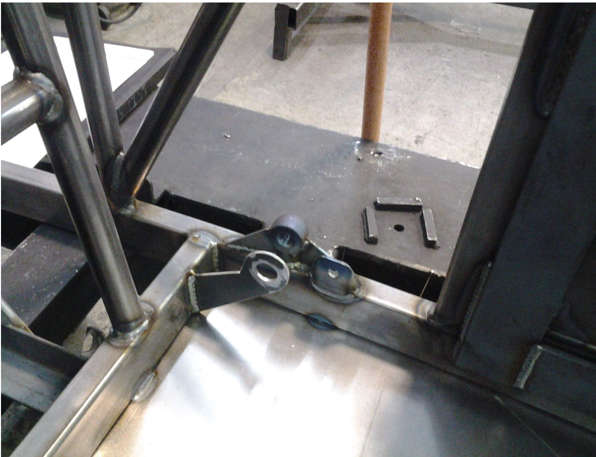
Taka-akselin alatukivarren tuplakorvakiinnike
