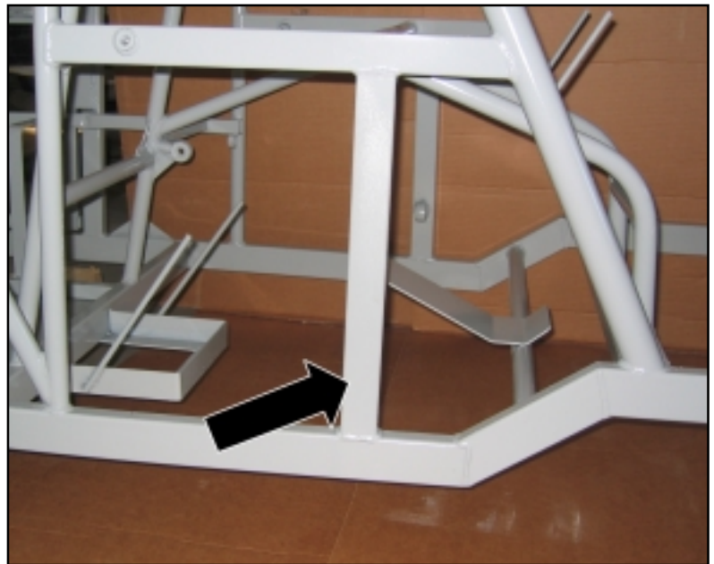
Pystytuki taka-akselikotelon takana suojaa polttoaine-tankkia jos taka-akselisto irtoaa.
