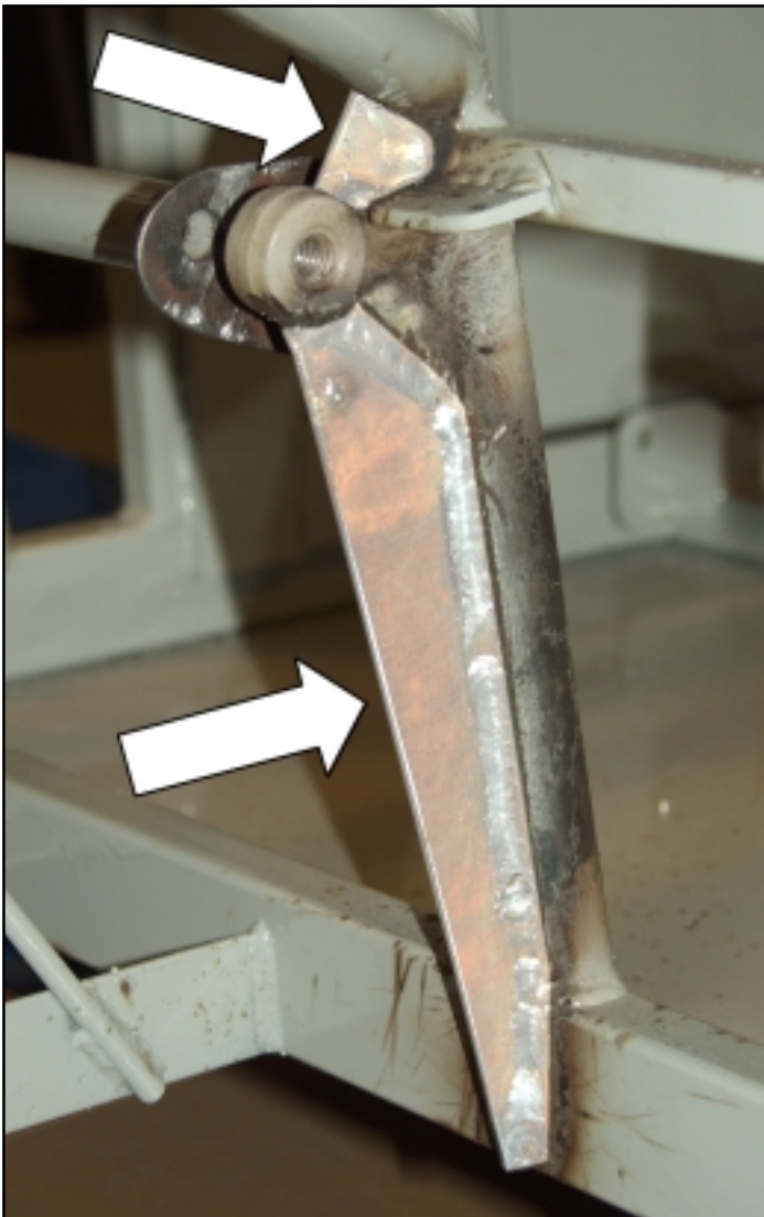
Ylälinkin kiinnityskorvan lisävahvikkeet. HUOM! Ei INEX-hyväksytty! Kansallinen lisäsääntö Suomessa.
