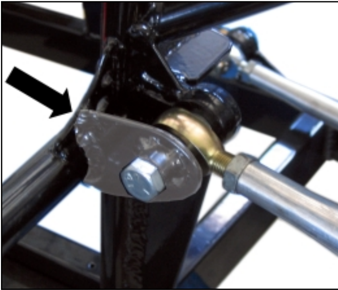
Ylälinkin tuplakorva, korin puoleinen
