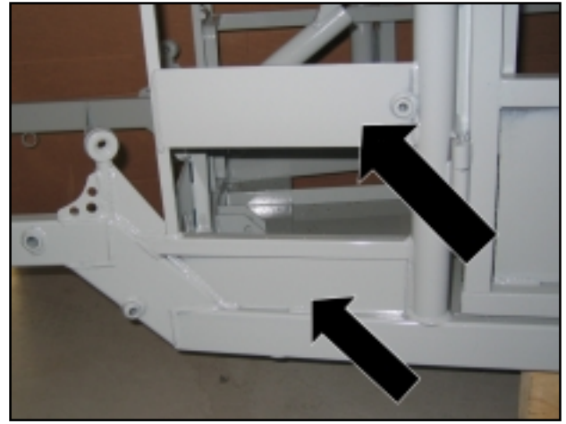
Paloseinän tukilevy, vasen (ylempi) Etuisan tukilevyt, vasen (alempi)
