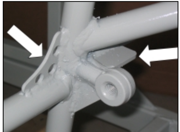
Ylälinkin kiinnityskorvan vahvikkeet, korin puoleiset.
