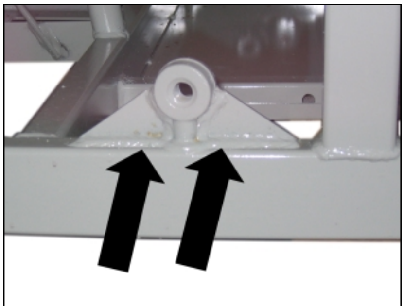
Takatukivarsien kiinnityskorvien lisävahvikkeet.
